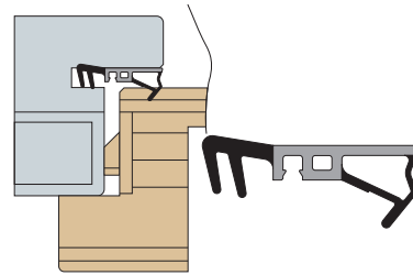
Das an der Zarge montierte Türprofil wurde aus zwei Komponenten (hartes PP (hellgrau) mit beidseitigen Dichtlippen aus flexiblem TPE) durch Coextrusion hergestellt.
