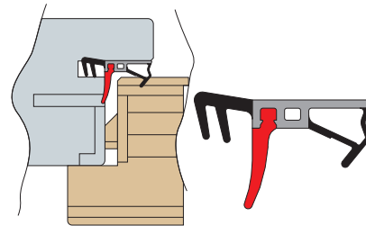
Hier wurde das gleiche Profil schon bei der Coextrusion mit einem zusätzlichen Streifen aus Fireblock versehen.
